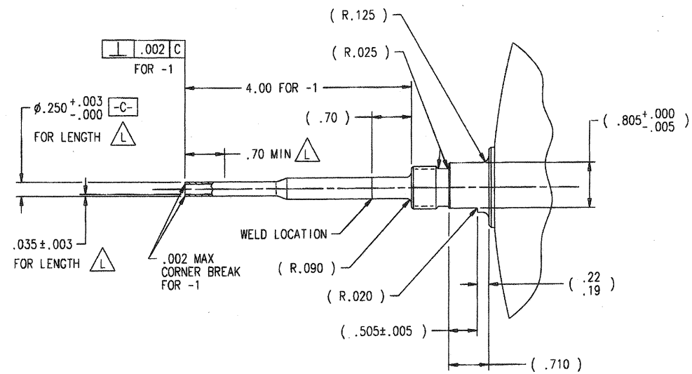
VIEW F-F SCALE: 1/1
